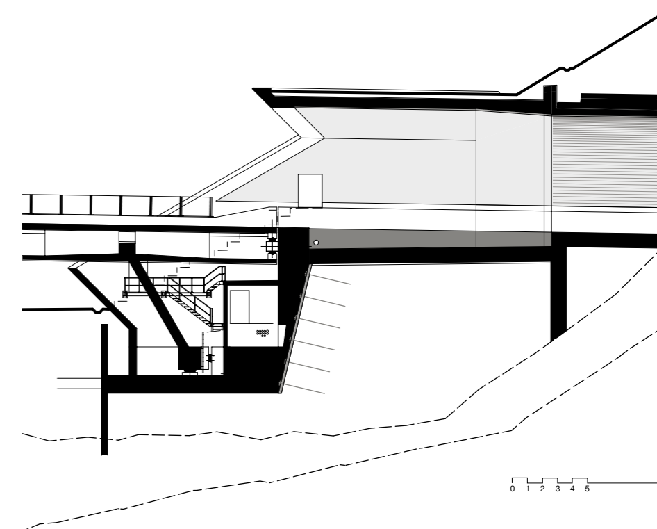
Längsschnitt durch die westliche Portalröhre / Coupe longitudinale à travers le tube ouest du portail
